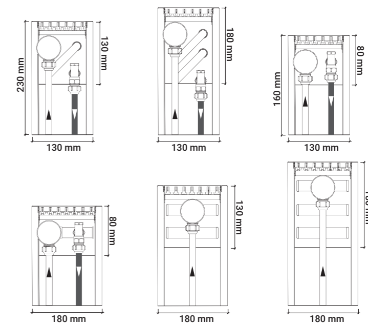
Типоразмерный ряд конвекторов Atrium Step
