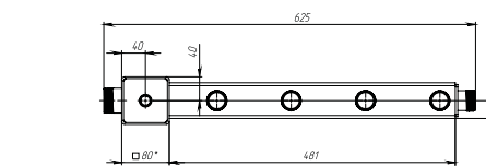
Блок коллекторный на 3(4) выхода, стрелка 60 кВт, AISI 304, артикул RTE 54.120
