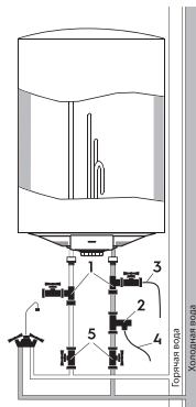
Рис. 4. Схема подключения к водопроводу моделей Nero
