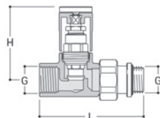
Вентиль Riapo прямой
